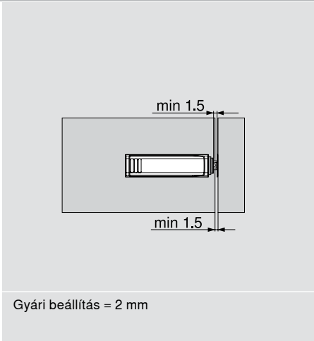
Egyenes adapterlemez
